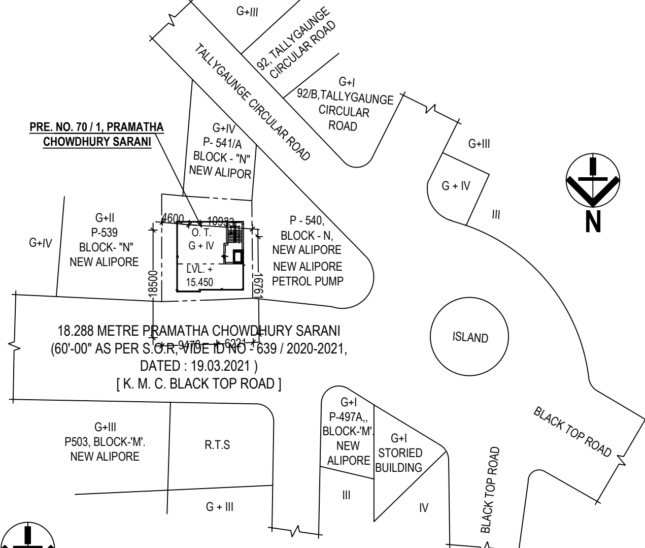
SITE PLAN SCALE - 1 : 600
